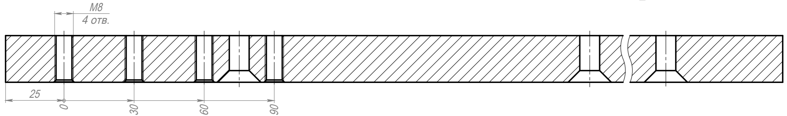
Б-Б (2 : 1)
