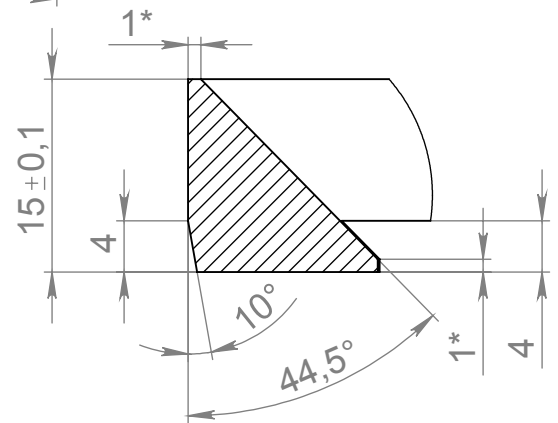
Б (2:1)
