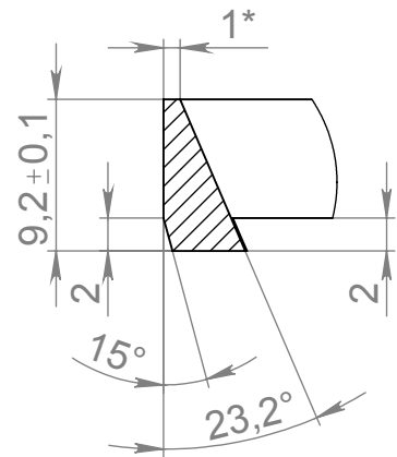
Б (2 : 1)
