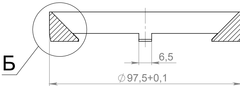
A-A (1:1)
