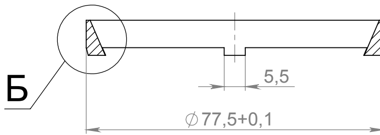
A-A (1 : 1)
