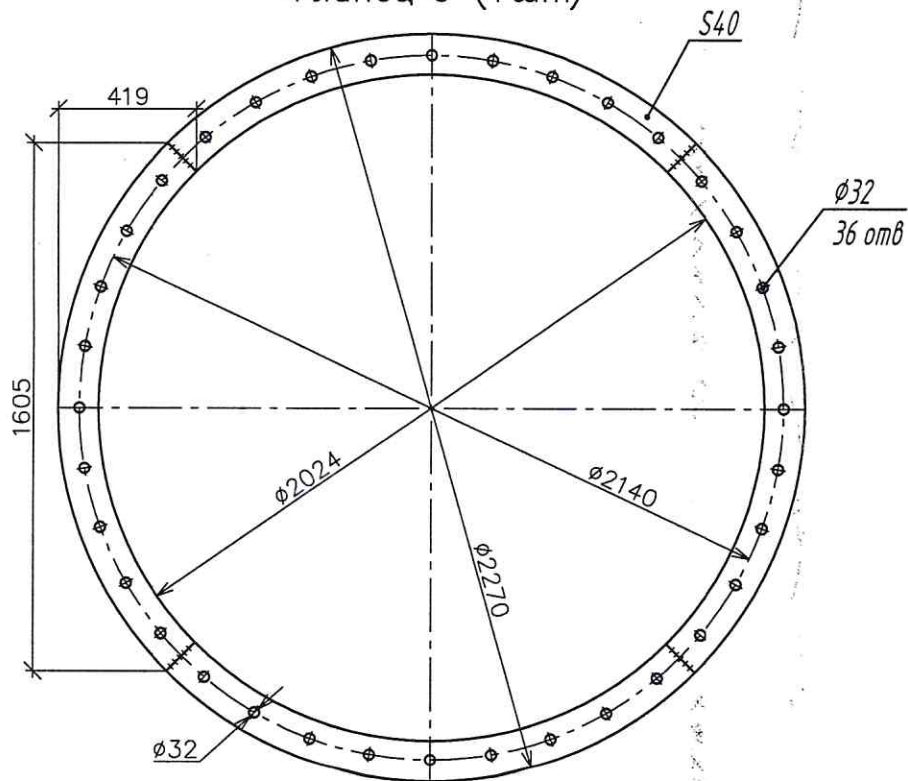
Фланец 6 (1 шт)
