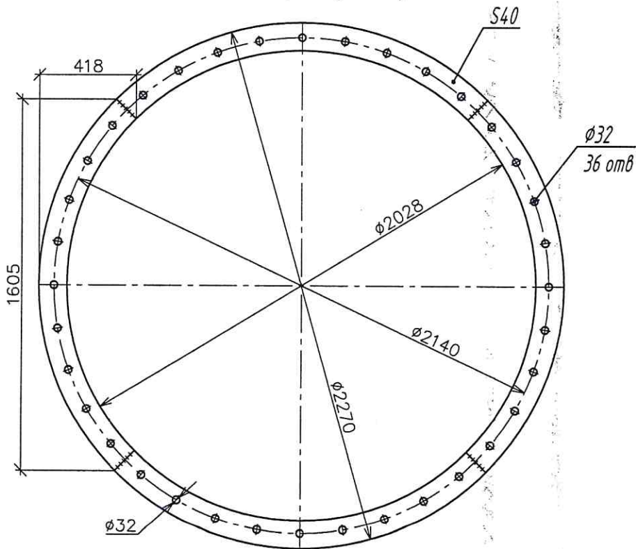
Фланец 4 (1 шт)
