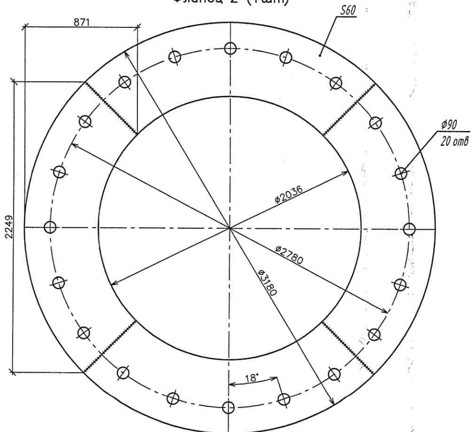
Фланец 2 (1 шт)
