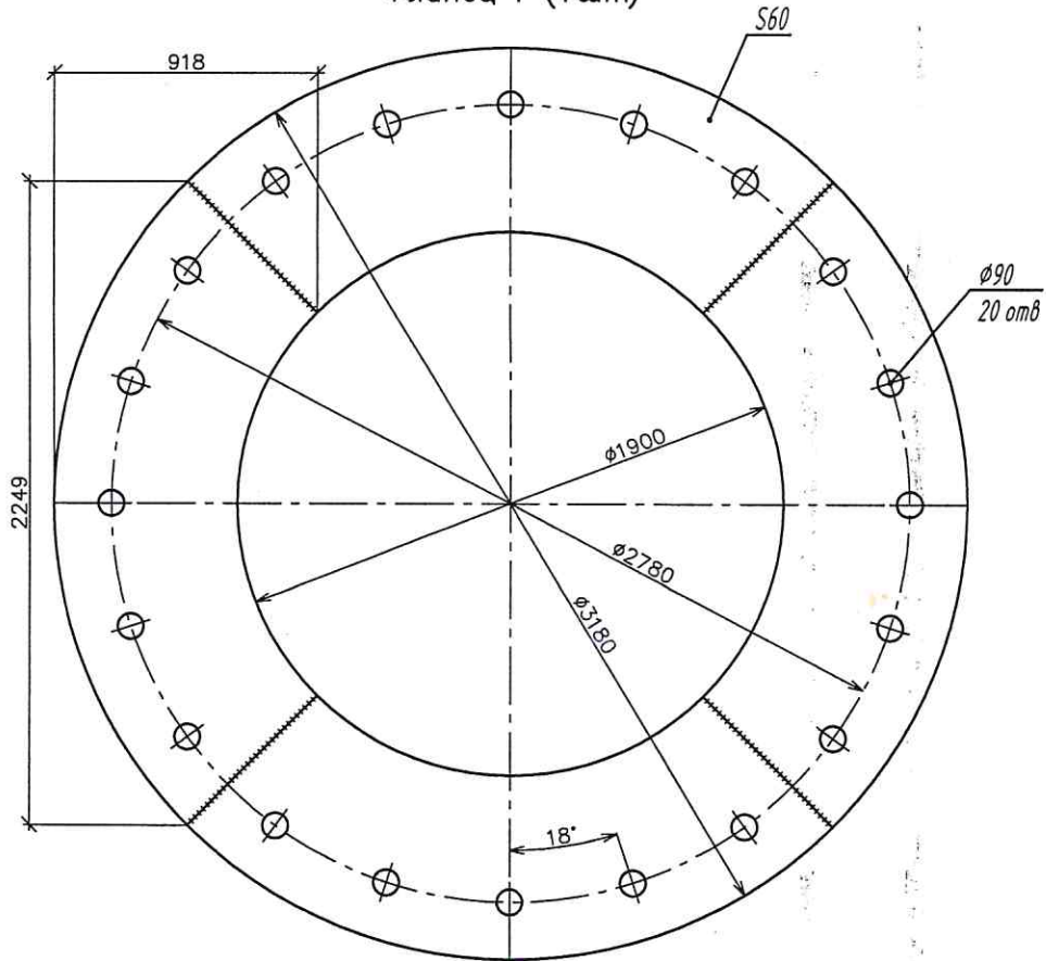
Фланец 1 (1 шт)
