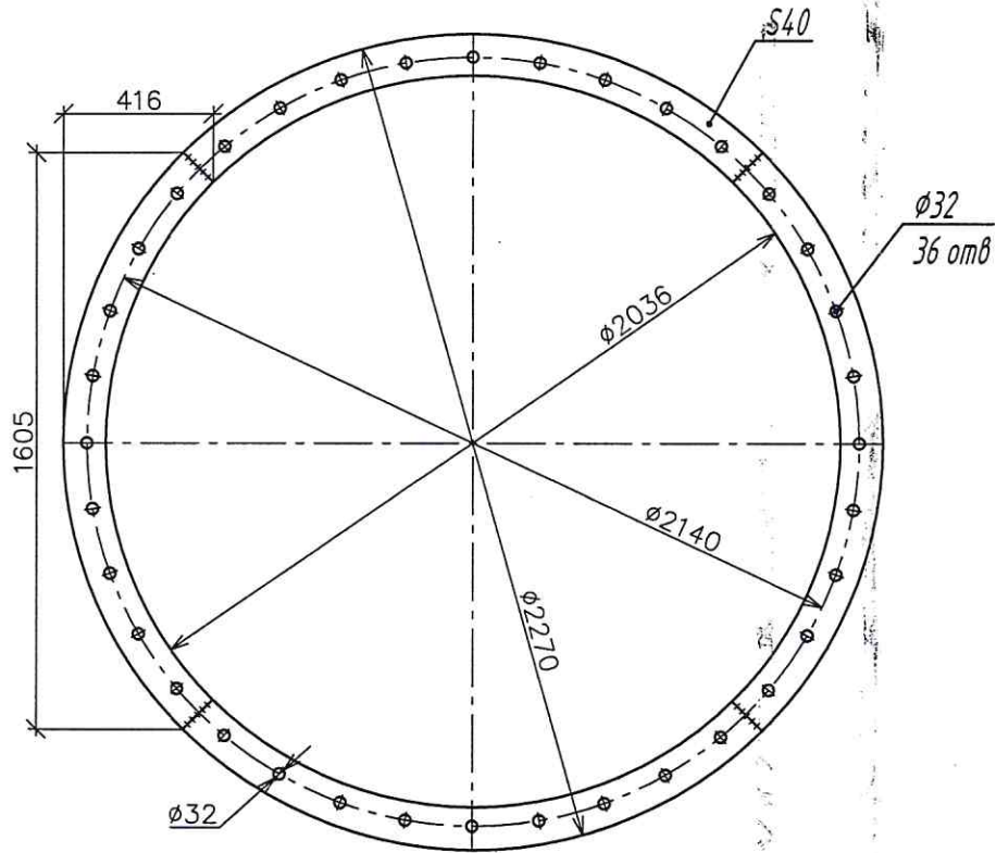
Фланец 3 (1 шт)
