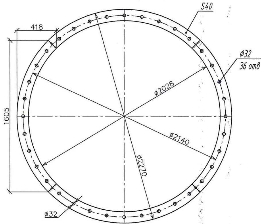
Фланец 5 (1 шт)
