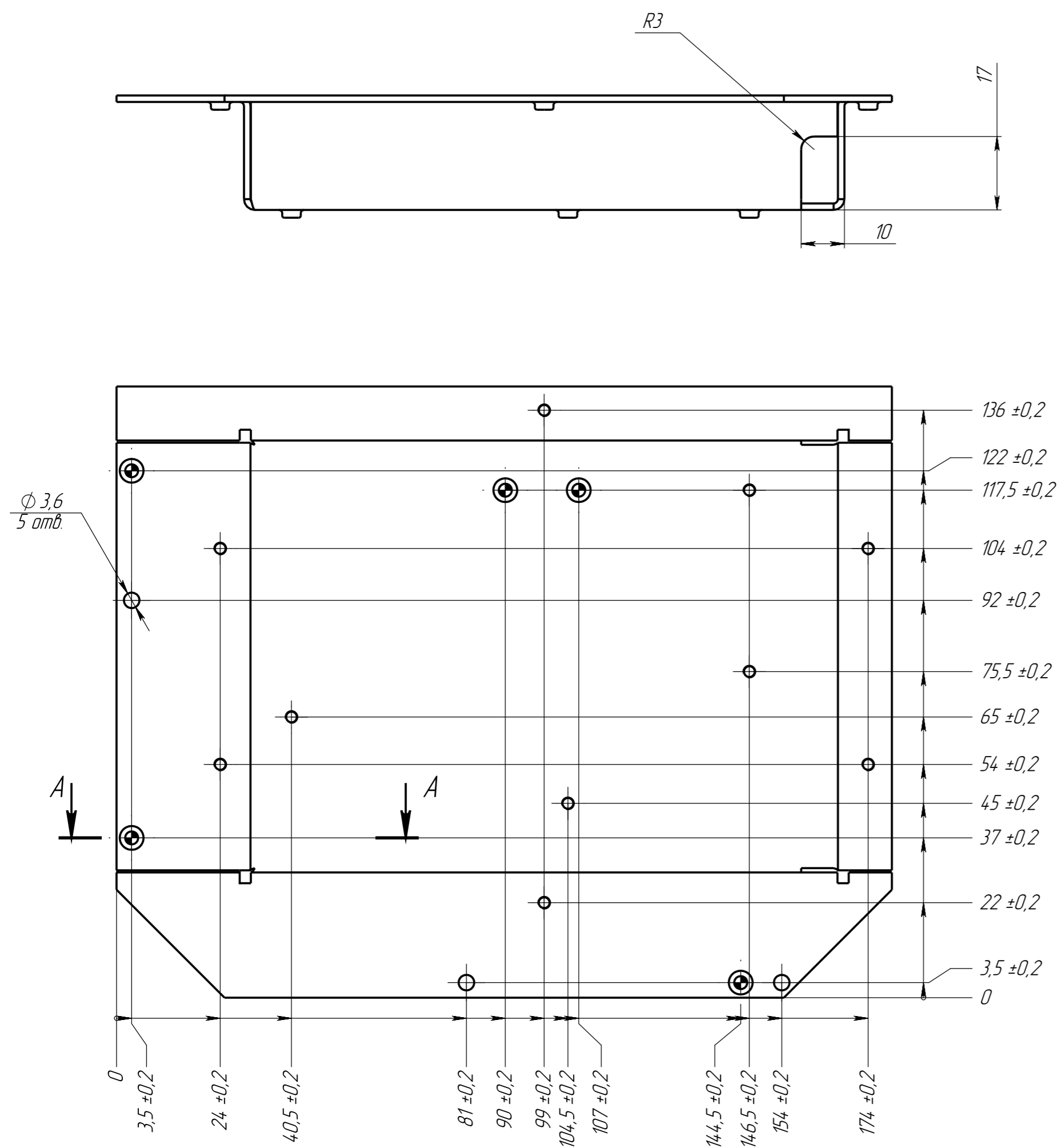
A-A (2 : 1)
