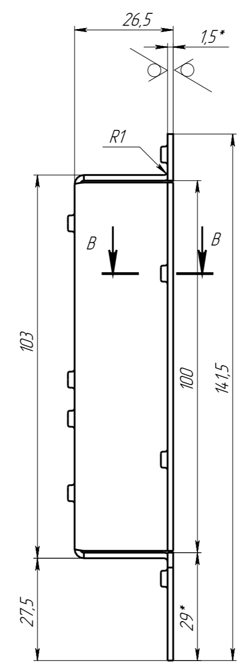
A-A (2 : 1)
