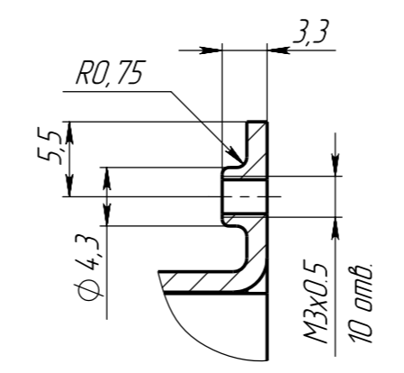
B-B (2 : 1)
