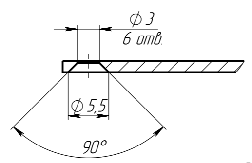
A-A (2 : 1)
