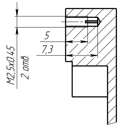
A-A (2 : 1)
