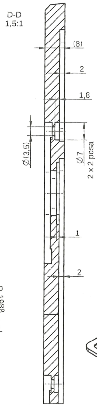
01.016 Верхняя пластина Материал: AL, 6082-T6 Лист: 2/3
