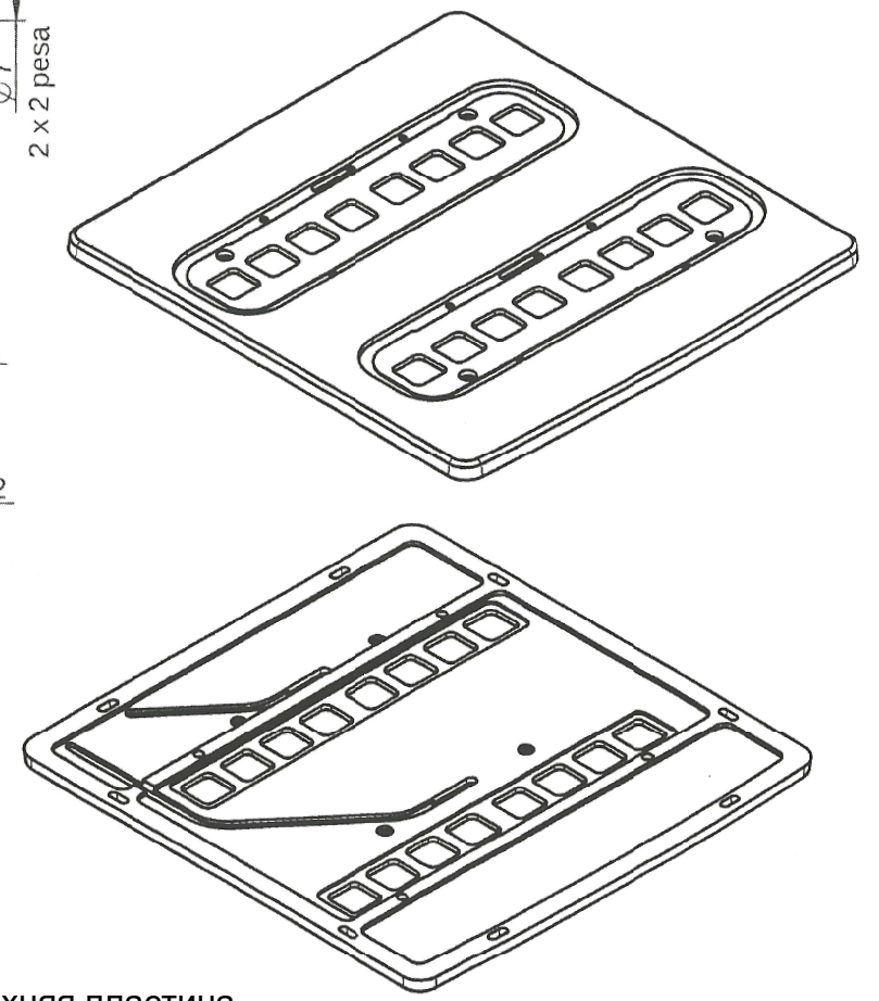
01.016 Верхняя пластина Материал: AL, 6082-T6 Лист: 2/3
