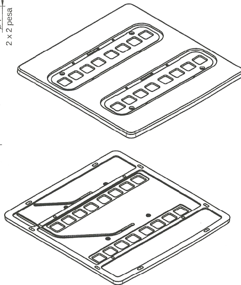
01.016 Верхняя пластина Материал: AL, 6082-T6 Лист: 2/3
