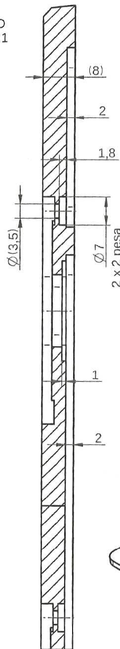
01.016 Верхняя пластина Материал: AL, 6082-T6 Лист: 2/3
