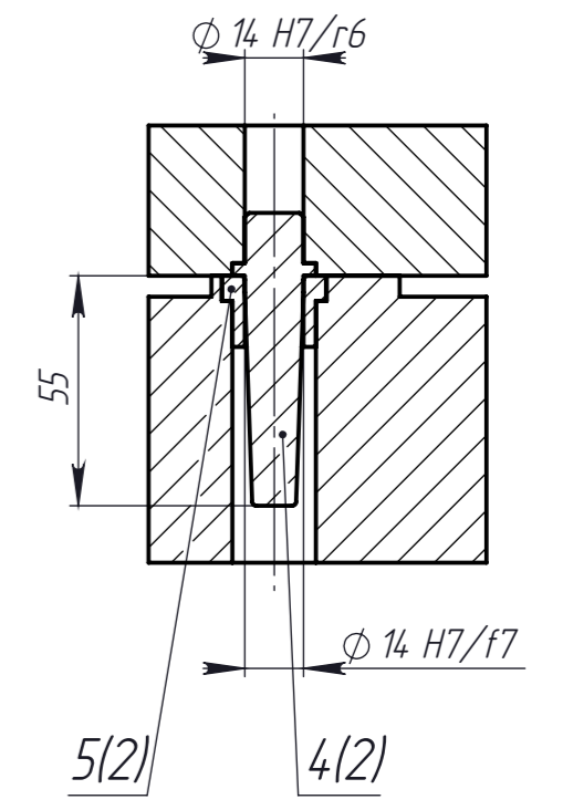
B-B (1:2)
