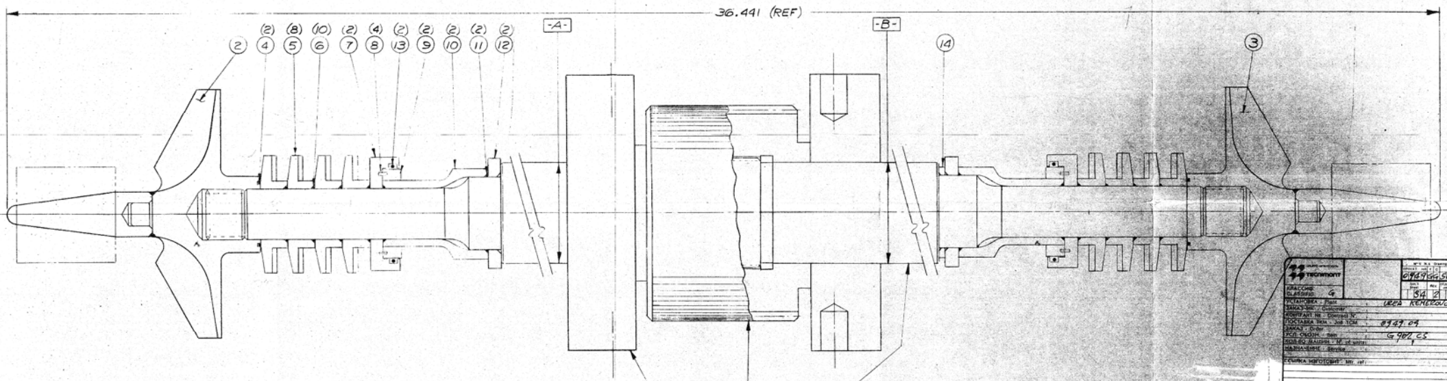
SH04HA05- (REF) SHAFT ASSY HI-SPEED вал высокой скорости
