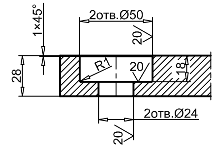
Б-Б M2:1
