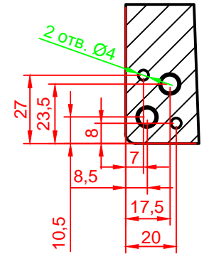
A-A (1:2)
