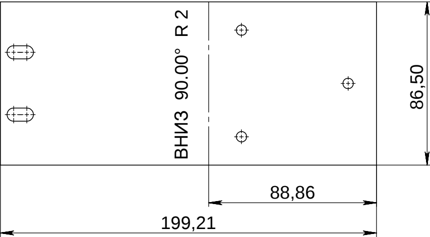
Развертка
