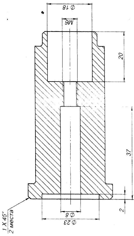
Рис.2 остальные размеры см. Рис.1
