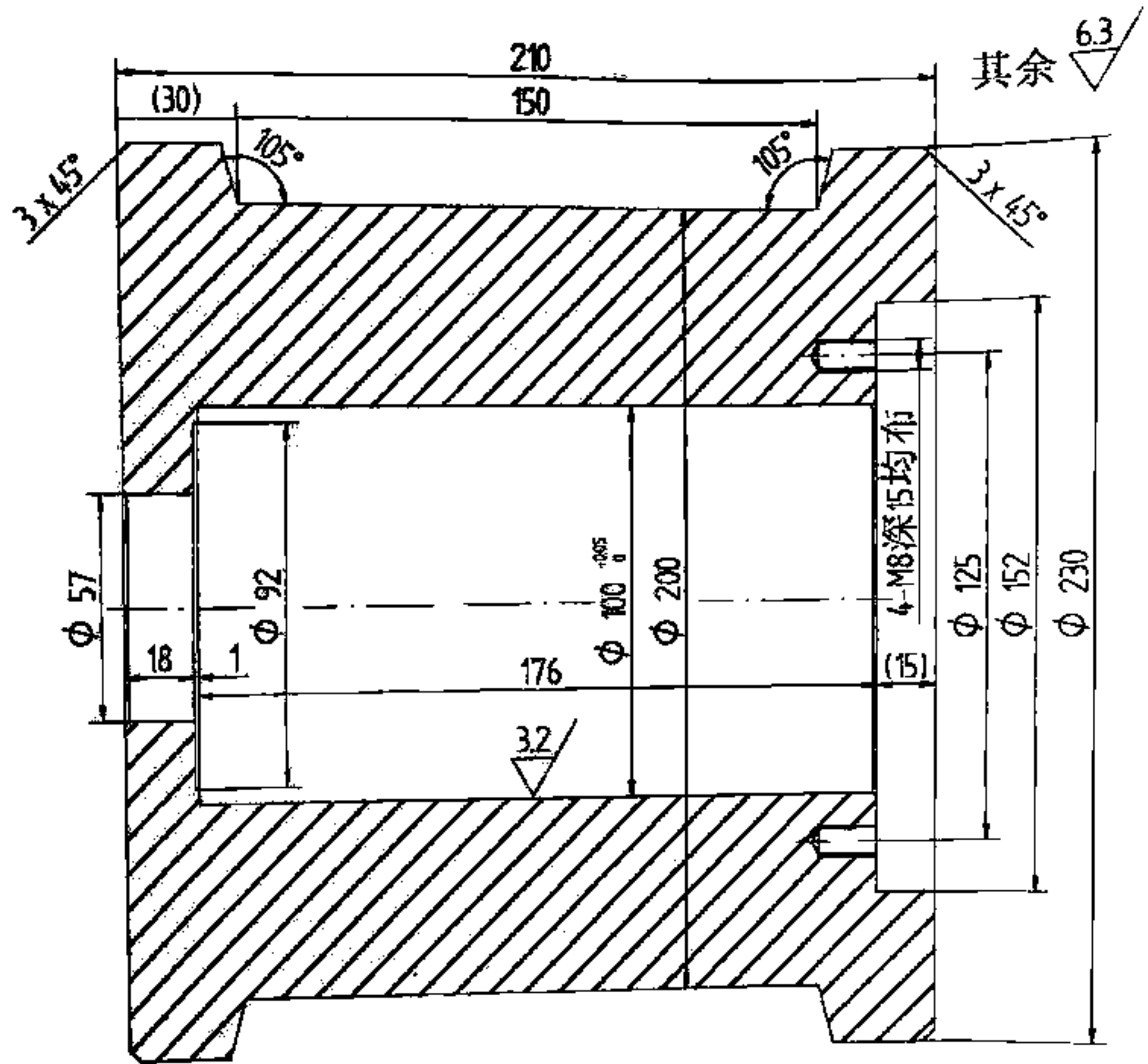
剖面 A-A
