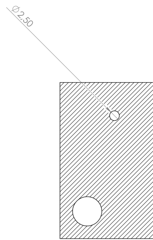
СЕЧЕНИЕ А-А
