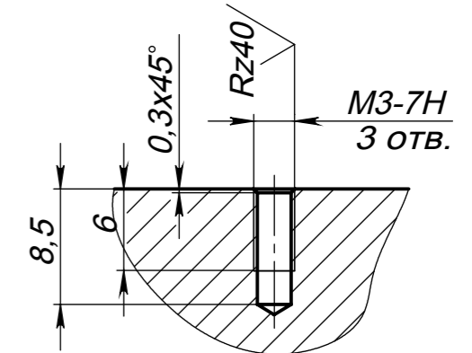
В-В (2:1)
