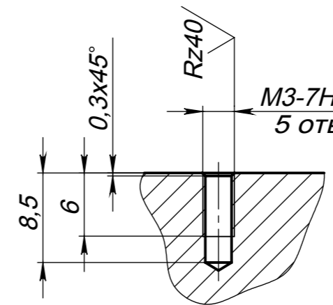
Г-Г (2:1)
