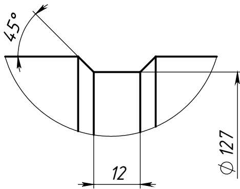
ВИД А (1 : 1) 2 канавки
