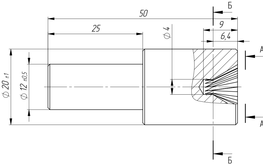
A-A (5 : 1)
