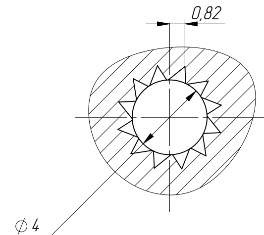
Б-Б (5 : 1)
