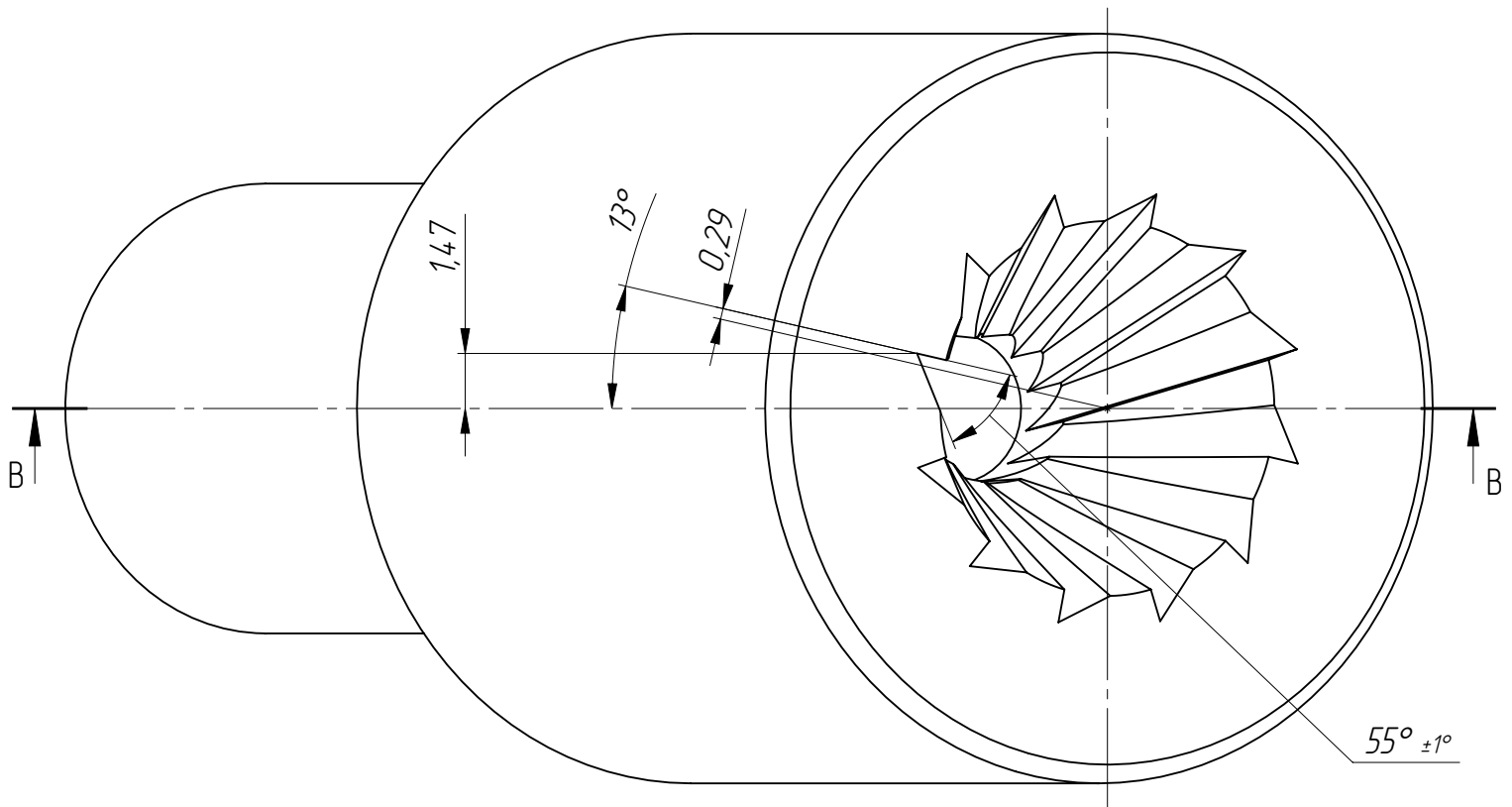
Вид перпендикулярно оси долбежного станка
