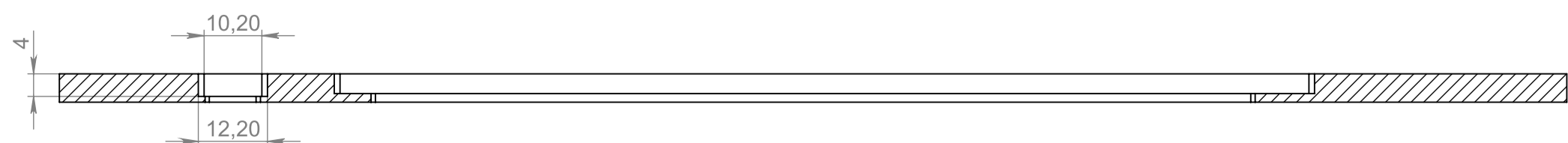
G-G
