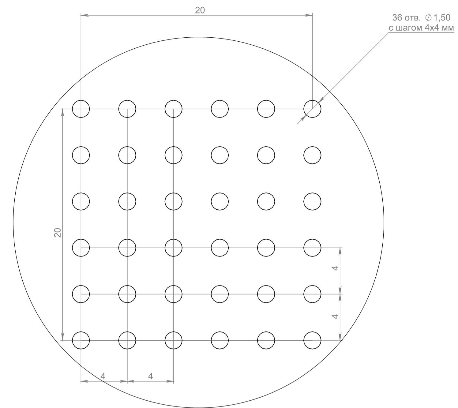
A (5 : 1)
