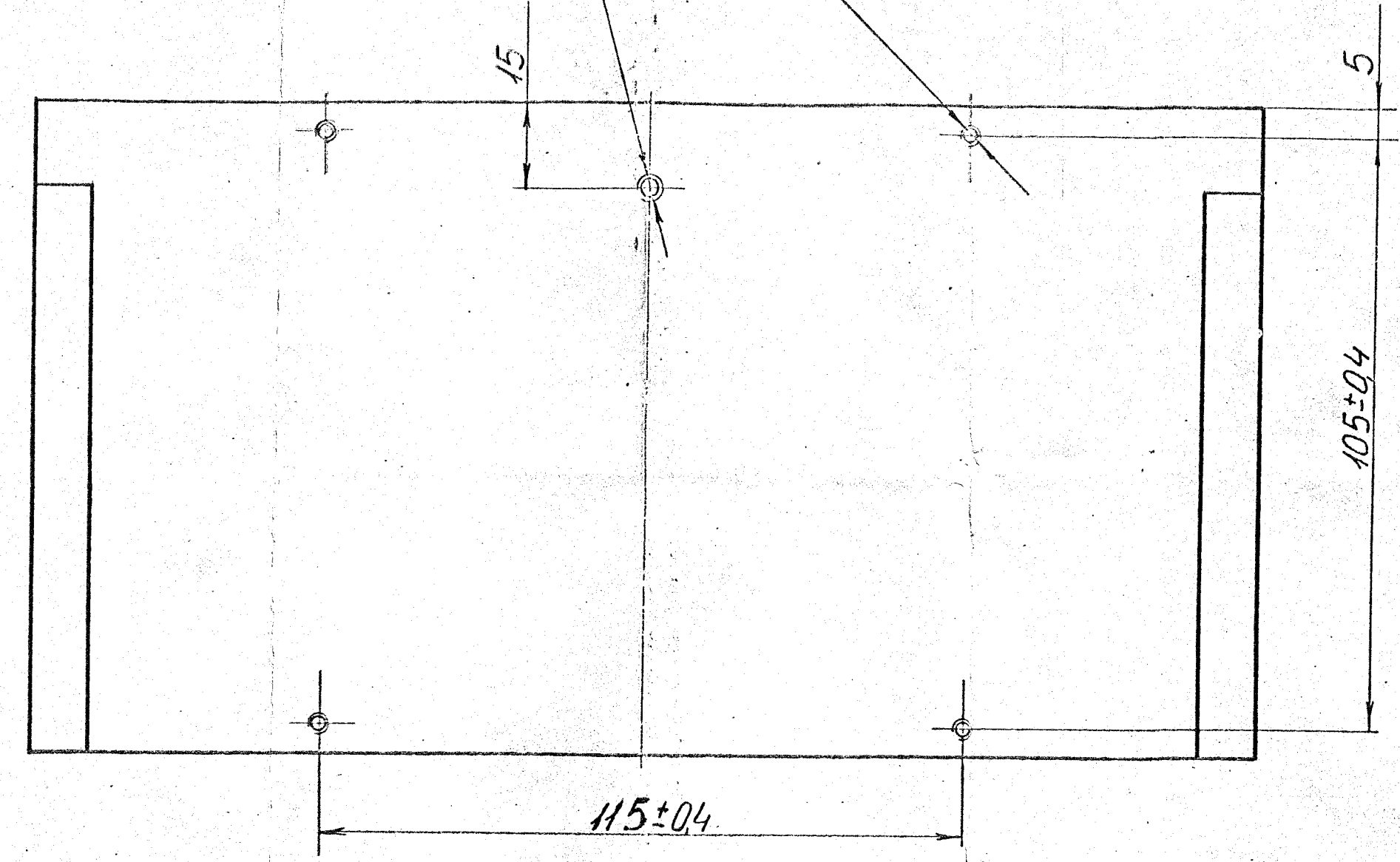
Вид А лист 1
