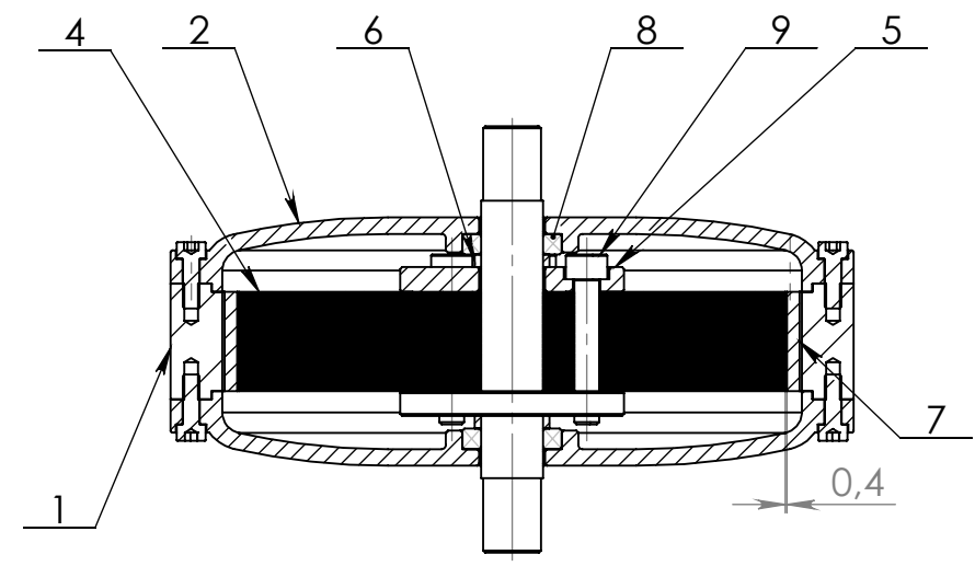
СЕЧЕНИЕ А-А
