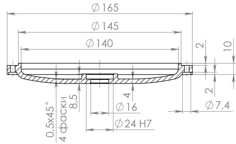
СЕЧЕНИЕ Е-Е
