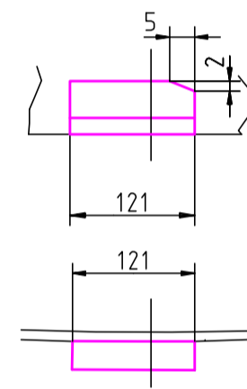
Зубец стандартный
