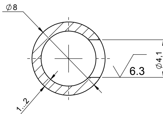
СЕЧЕНИЕ А-А 4 : 1
