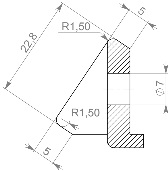
A-A (2 : 1)
