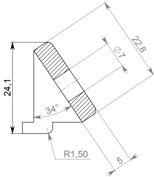
B-B (2 : 1)
