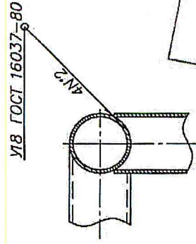
Б (1:1)
