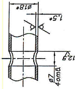
A-A (1:1)
