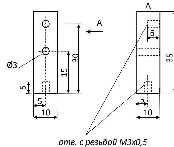
Стойка №2 (16 шт.), материал -сталь
