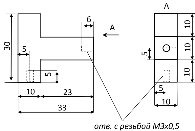
Стойка №1 (16 шт.), материал -сталь
