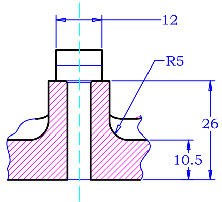
Б-Б (1:1)
